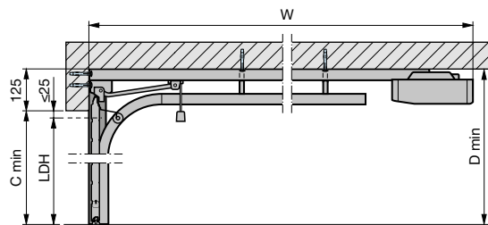
Vertikalsnitt
